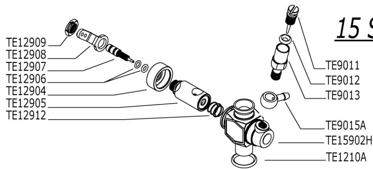
ROTOR CARBURETOR
